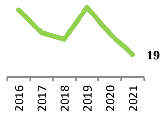
Üretim (GW/h)
