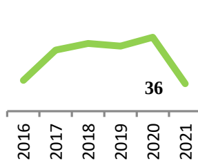
Üretim (GW/h)
