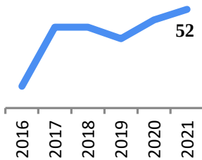
Üretim (GW/h)
