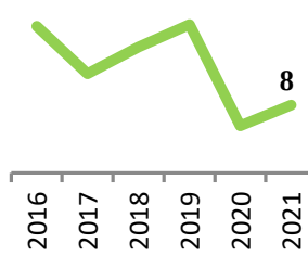
Üretim (GW/h)
