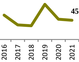
Üretim (GW/h)
