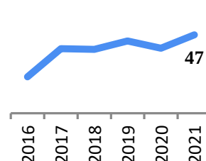
Üretim (GW/h)
