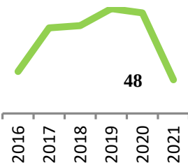
Üretim (GW/h)
